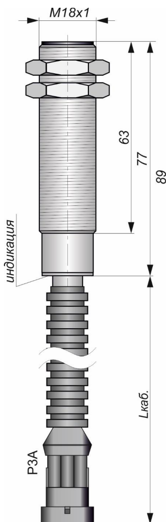
Габаритный чертеж
